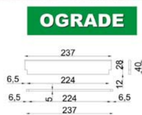
LIVENA ZIDNA PLATNA
